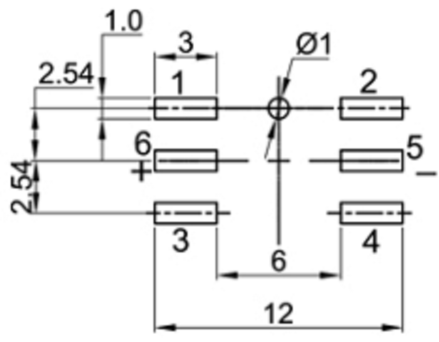
P.C.B. LAYOUT
