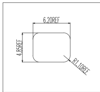
面板开孔参考尺寸
