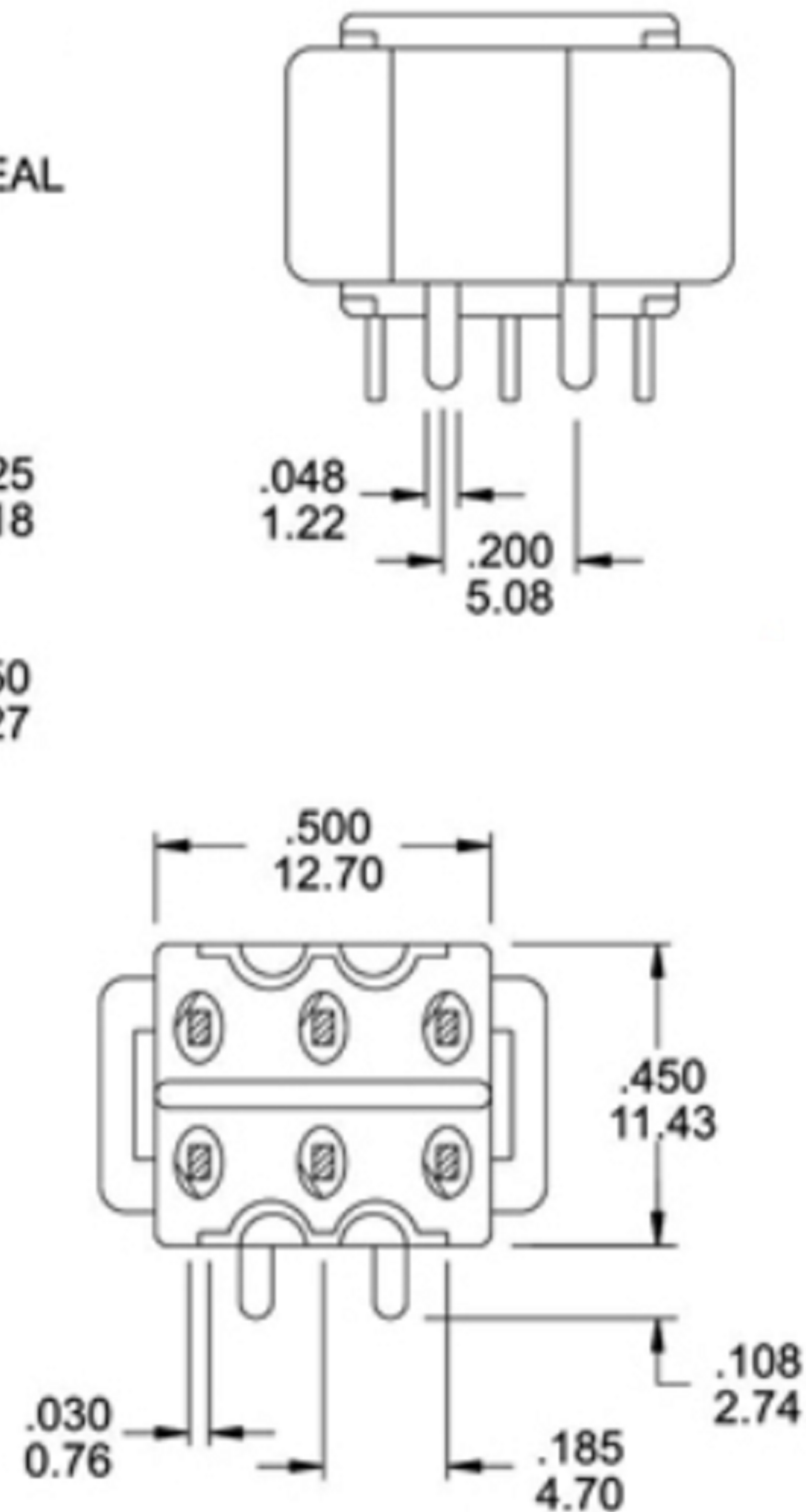
SECTION A-A
