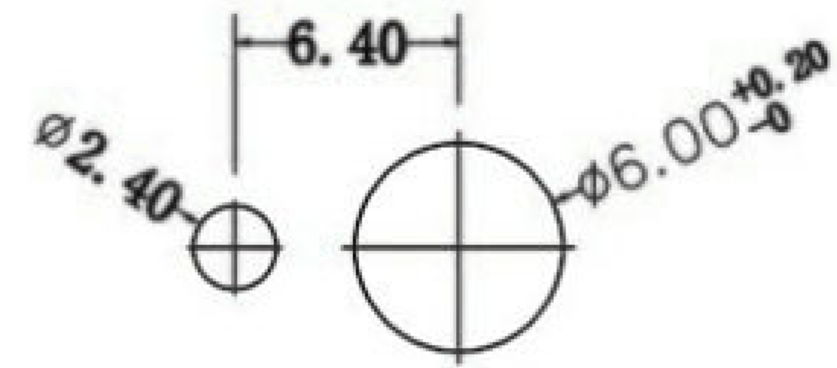
安装孔尺寸
