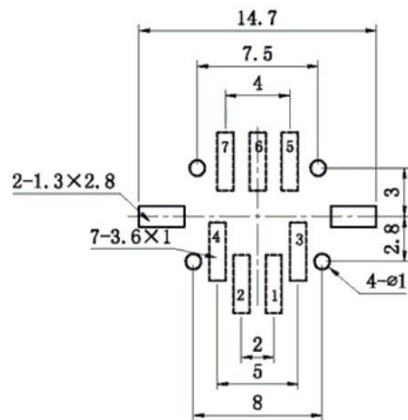
PCB板安装孔图
