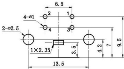
PCB板安装孔图
