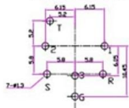
印制线路板示意图
