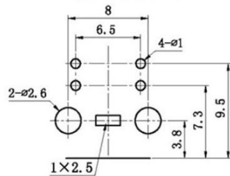
PCB板安装孔图
