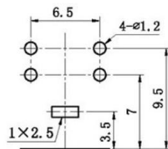
PCB板安装孔图
