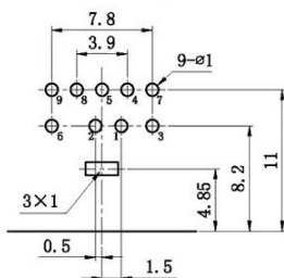
PCB板安装孔图
