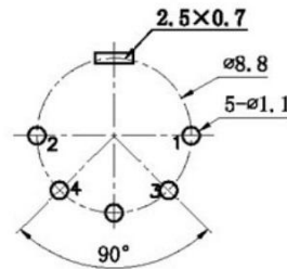
PCB板安装孔图
