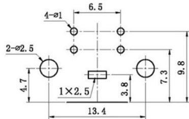
PCB板安装孔图
