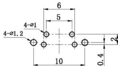
※ PCB板安装孔图
