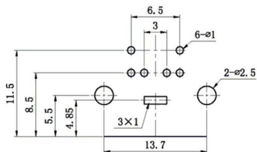
PCB板安装孔图
