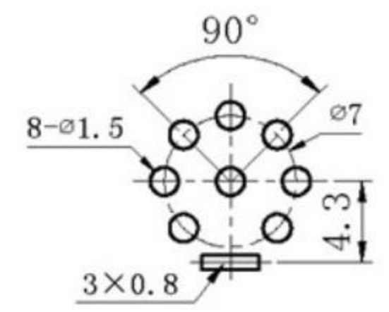
PCB板安装孔图
