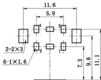
PCB板安装孔图
