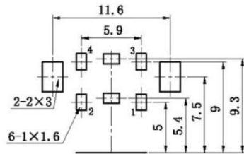
PCB板安装孔图
