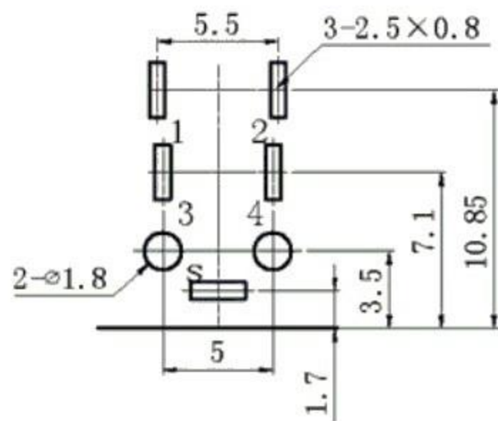
PCB板安装孔图
