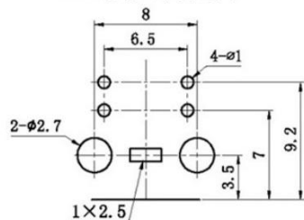
PCB板安装孔图
