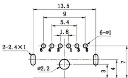
PCB板安装孔图
