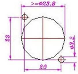
Frontblettenschnitt (Frontseite) Panel cut out (front side)
