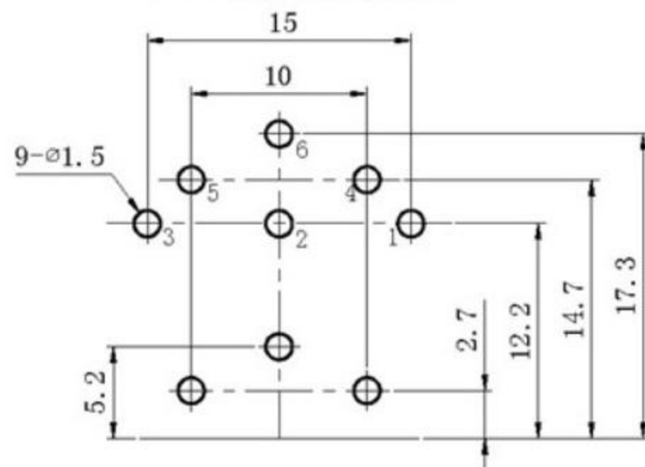
PCB板安装孔图
