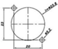
Frontlattenausschnitt (Frontseite) Panel cut out (front side)
