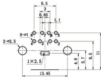
PCB板安装孔图
