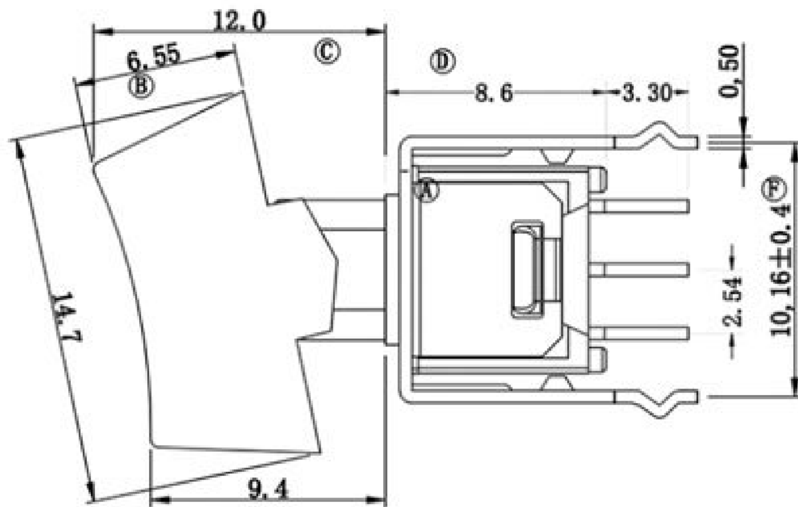
标注: ① - ⑥ 尺寸的重点检验尺寸
