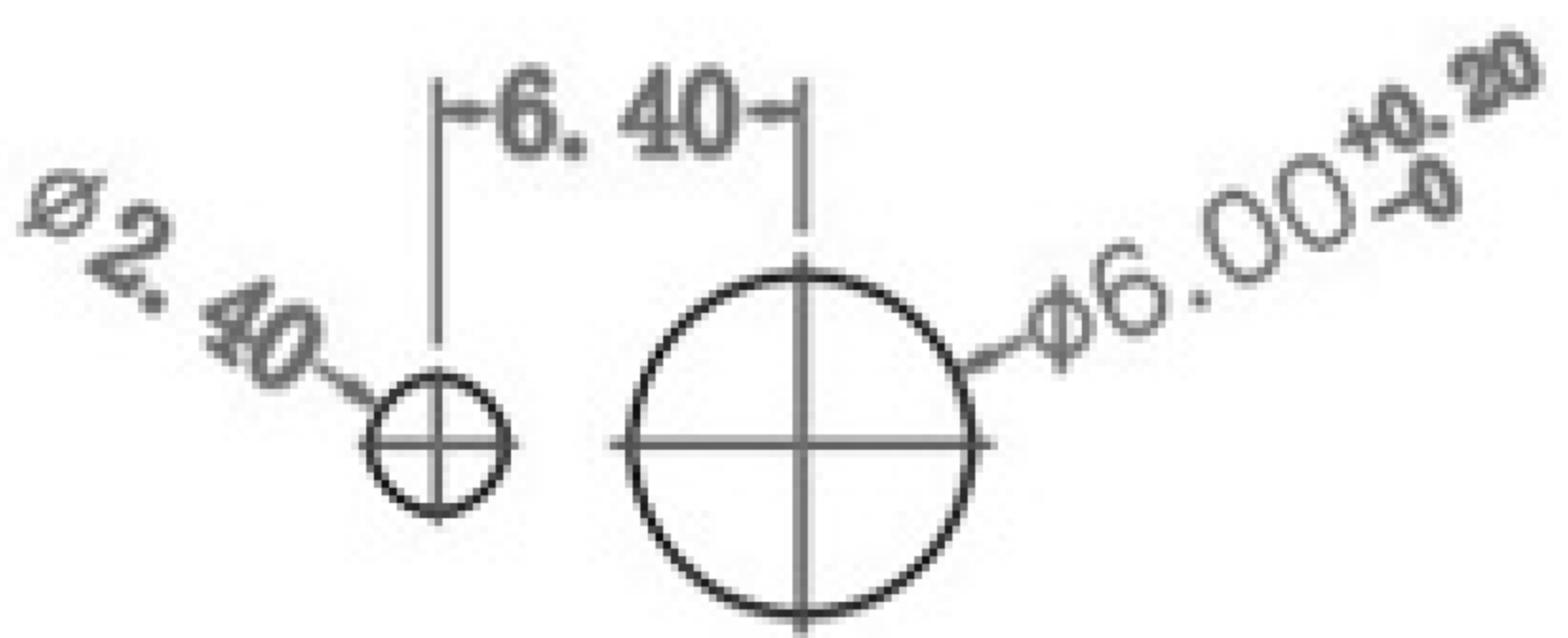
安装孔尺寸
