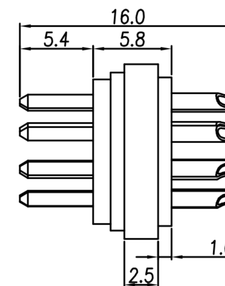
12PIN尺寸
