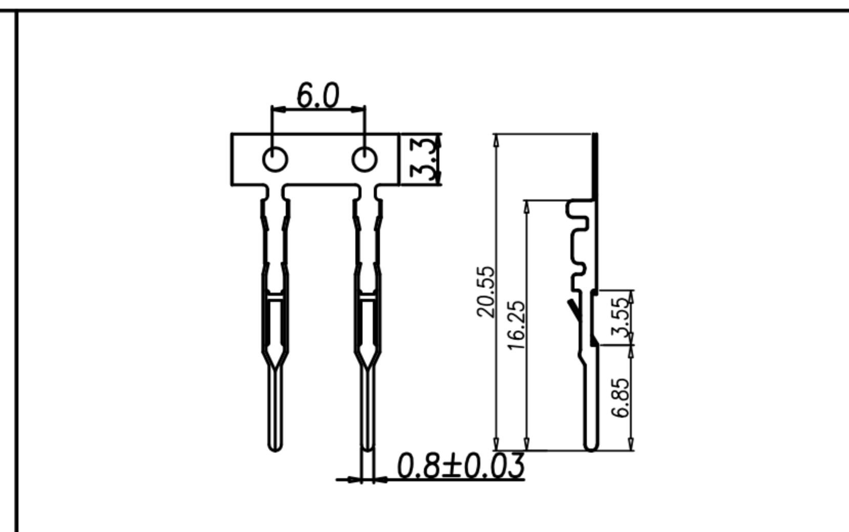
DY-DM0240(CONTACT)
