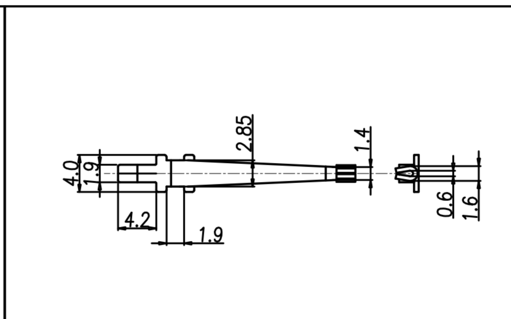
DY-DM0037(CLASP)
