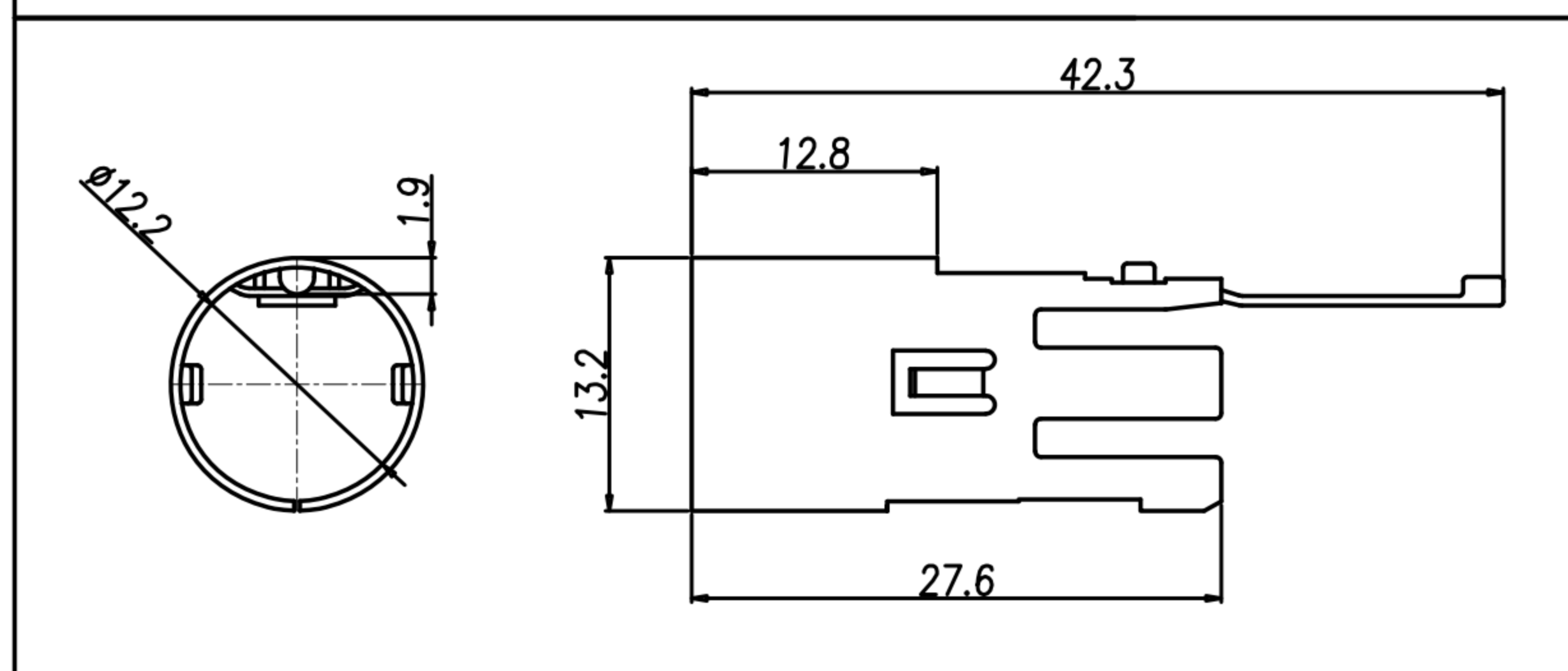
DY-DM0035(SHELL)
