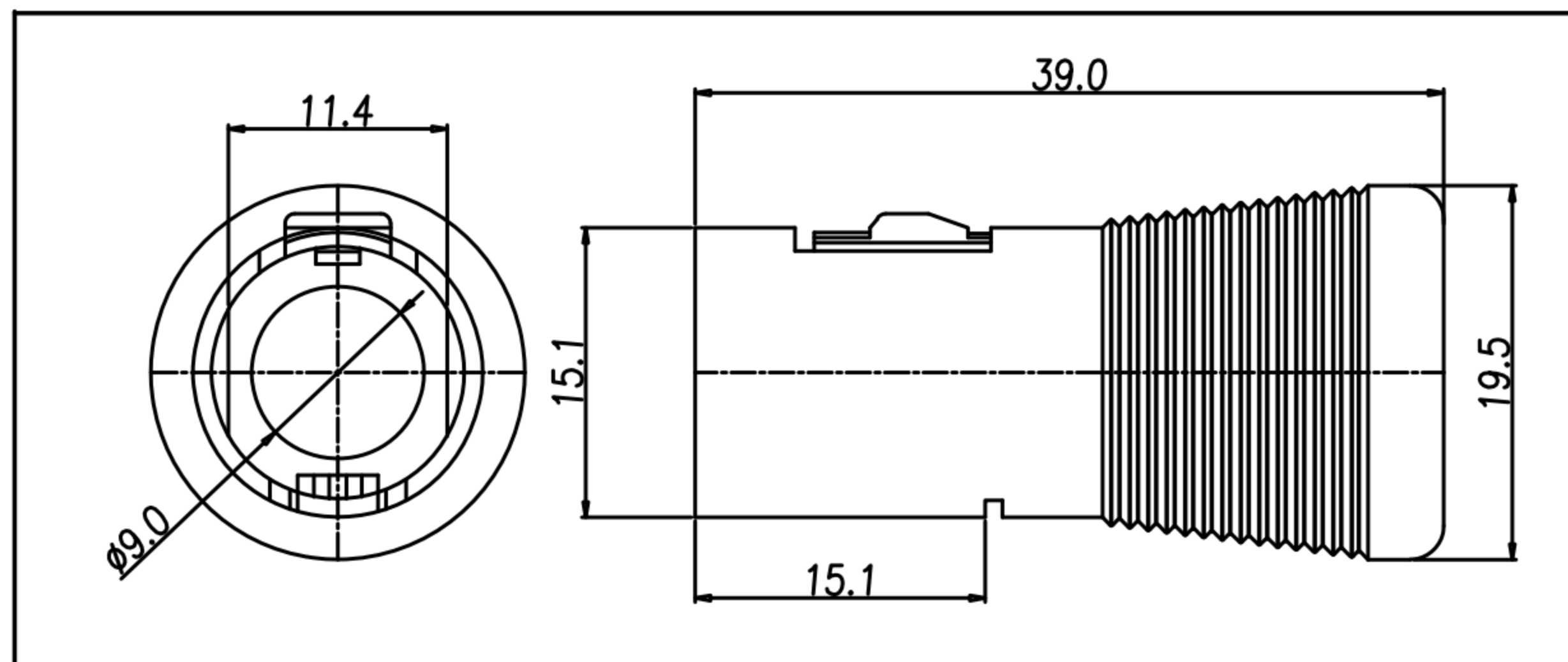
DN-DM0022(COAT)
