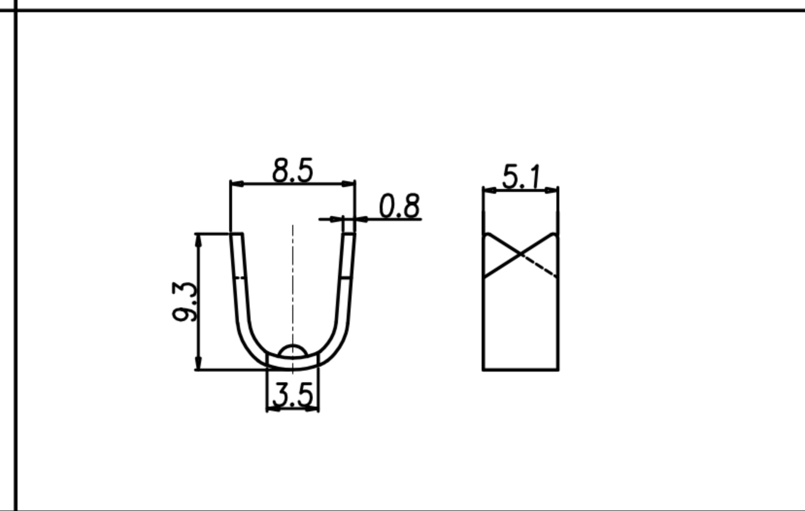
DY-DM0006(LINE BUCKLE)
