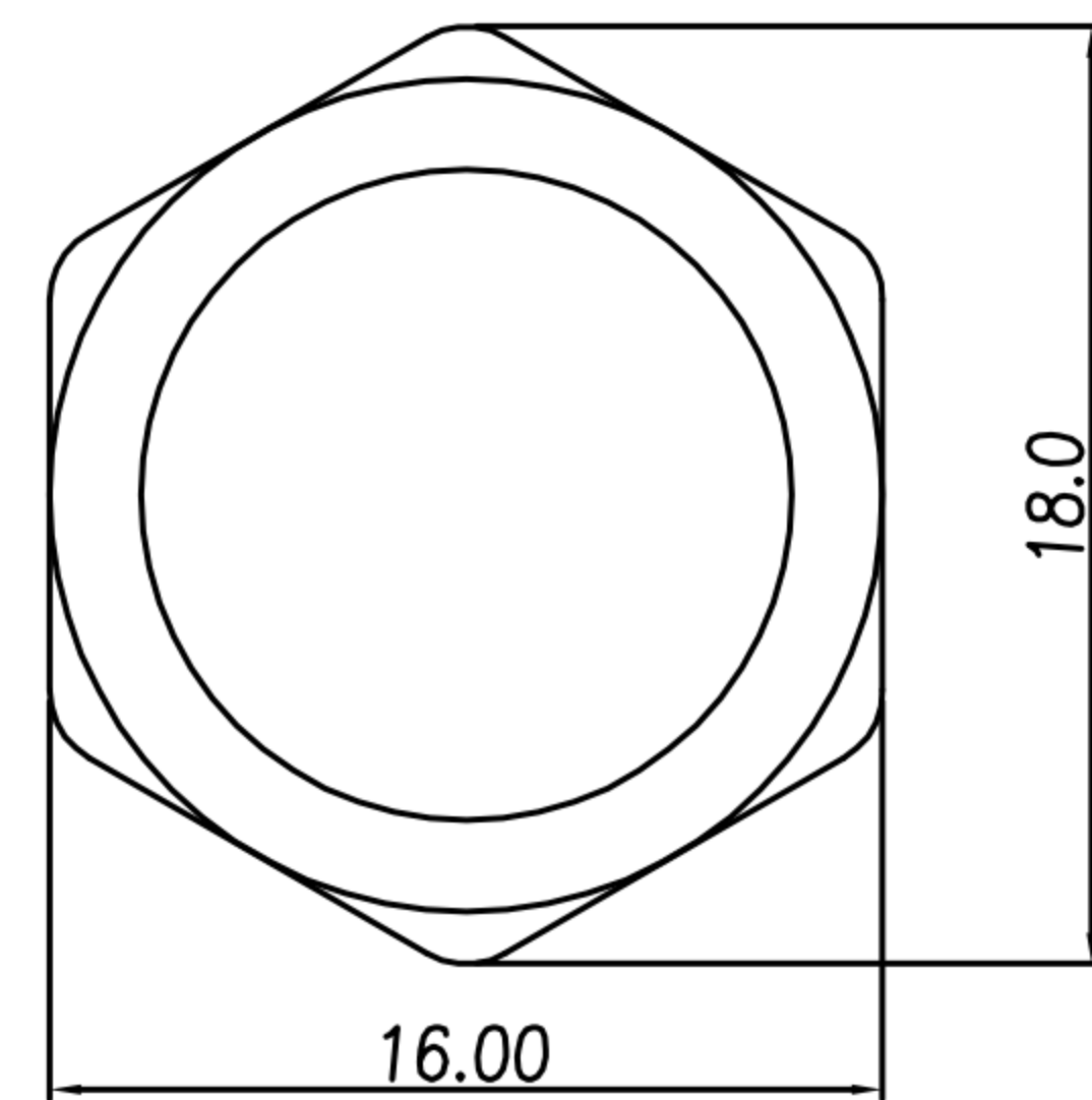
NUT
