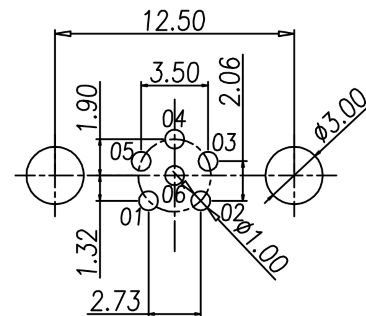
P.C.B LAYOUT
