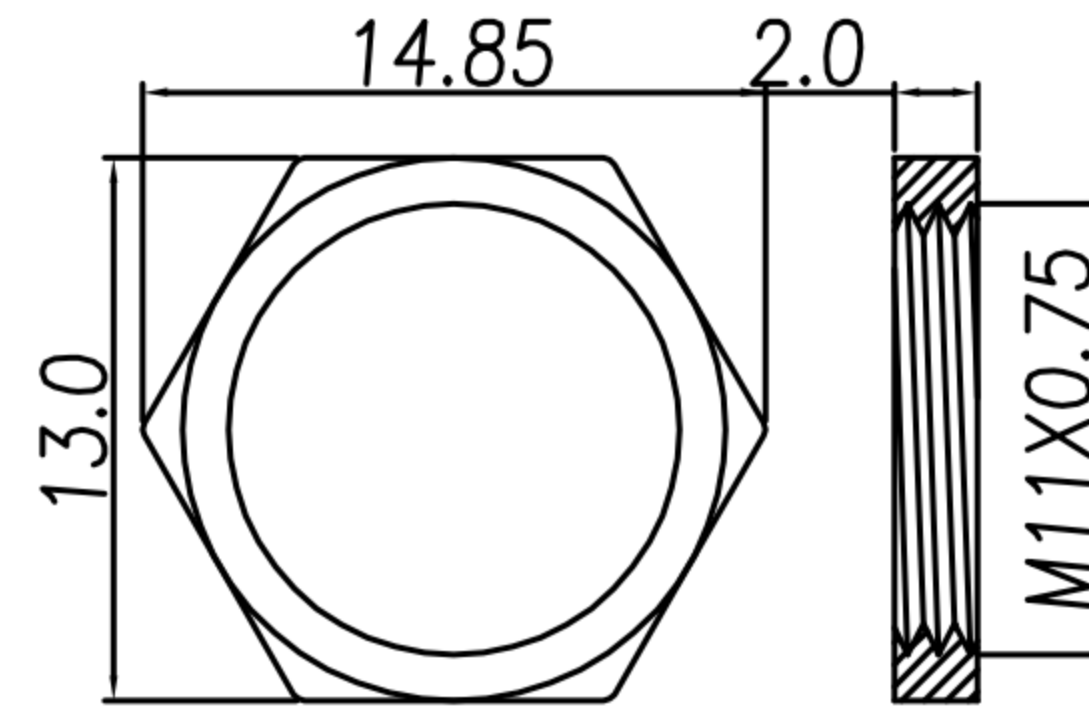
NUT
