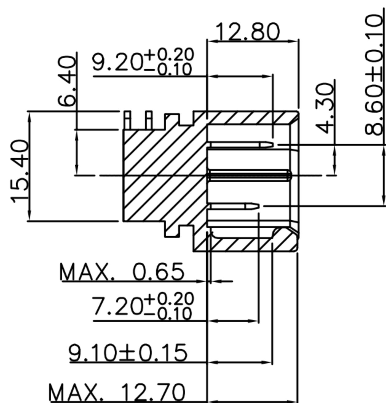
Section A-A(SCALE 1:1)
