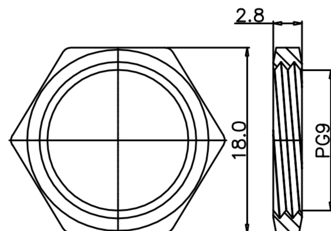
NUT
