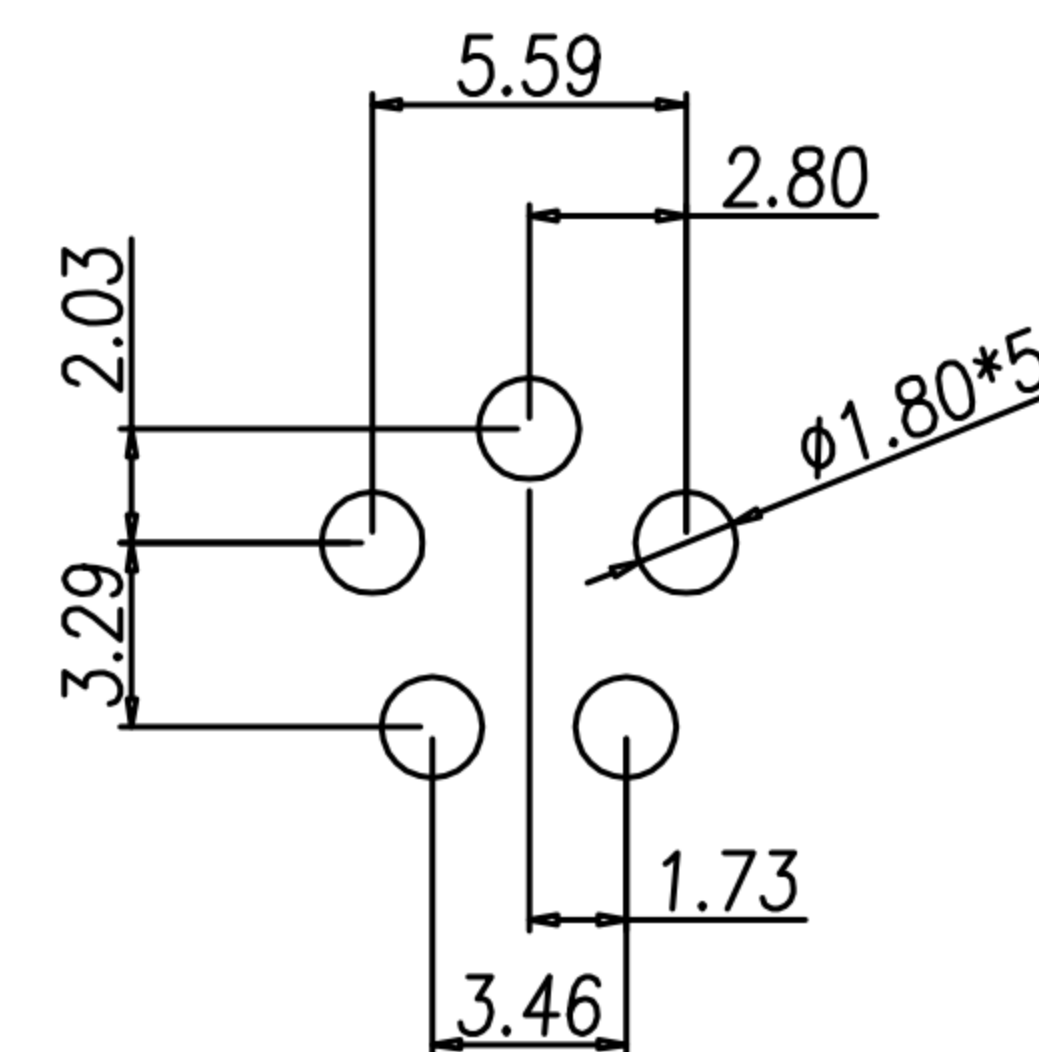
P.C.B LAYOUT
