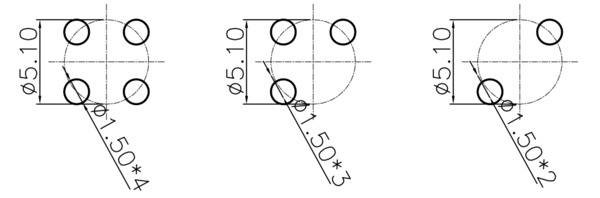
P.C.B LAYOUT
