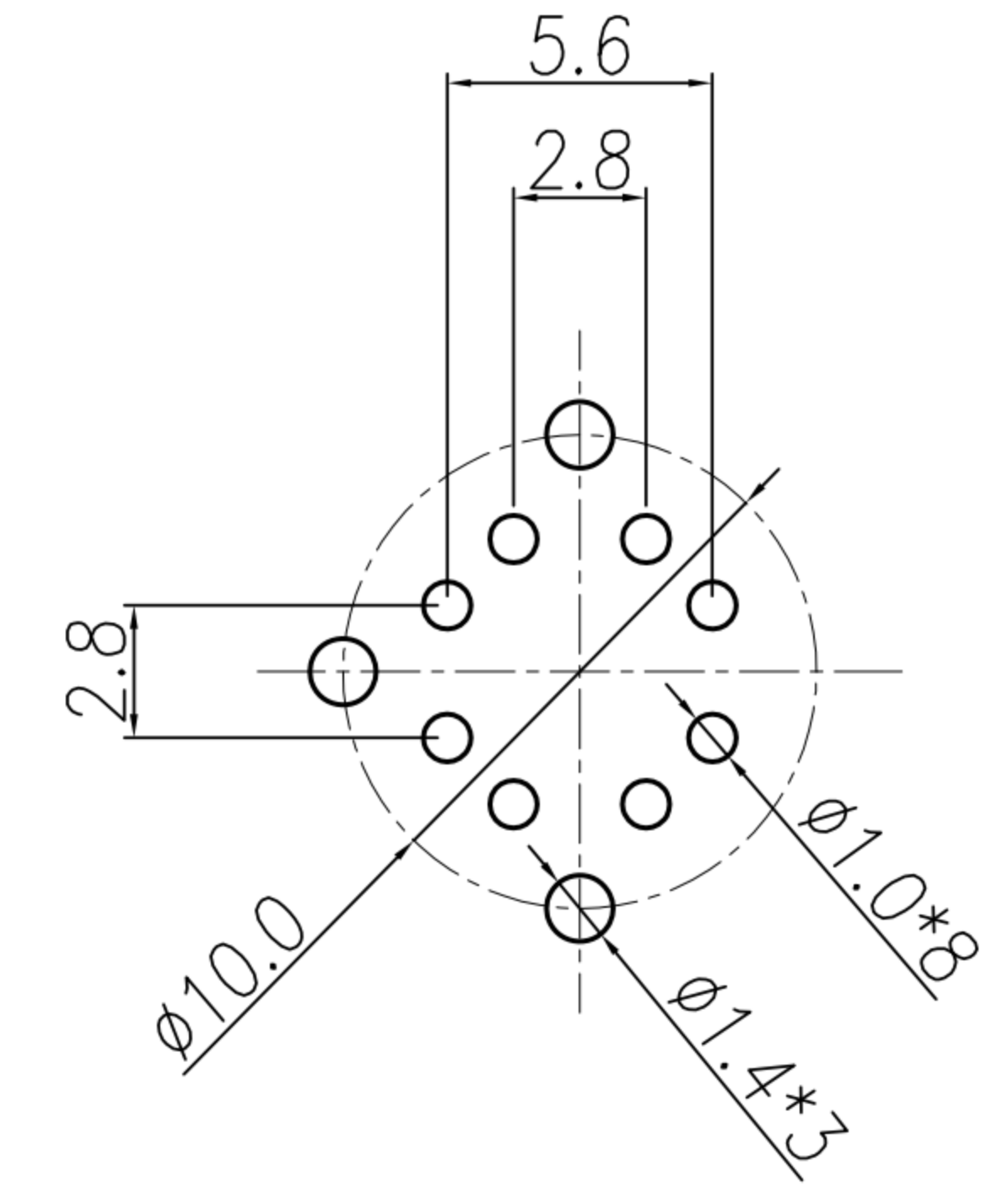
RECOMMEND P.C.B LAYOUT
