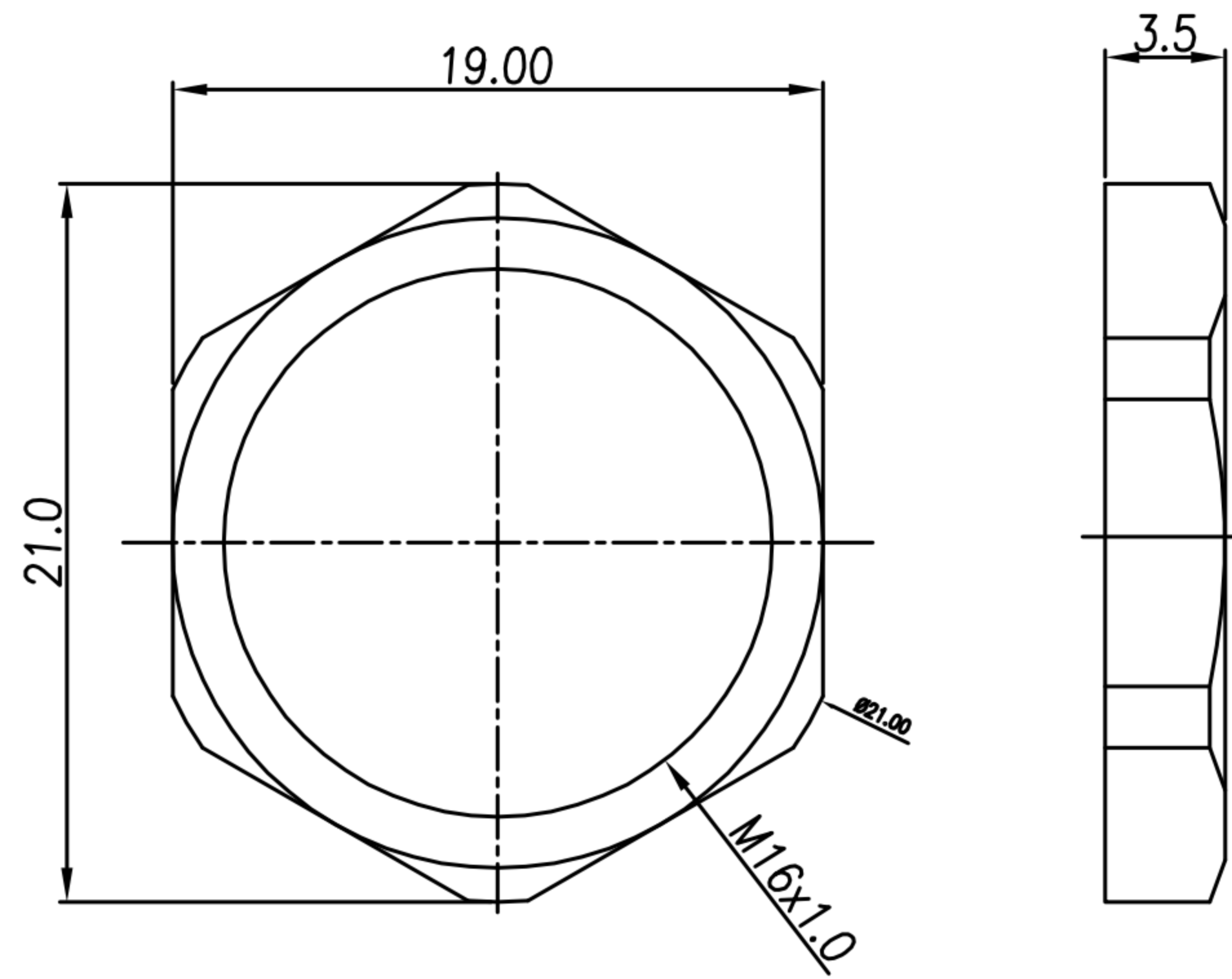
NUT
